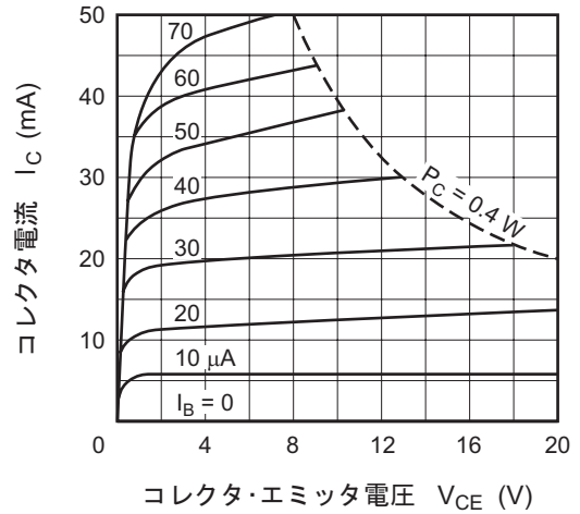
エミッタ接地出力静特性
