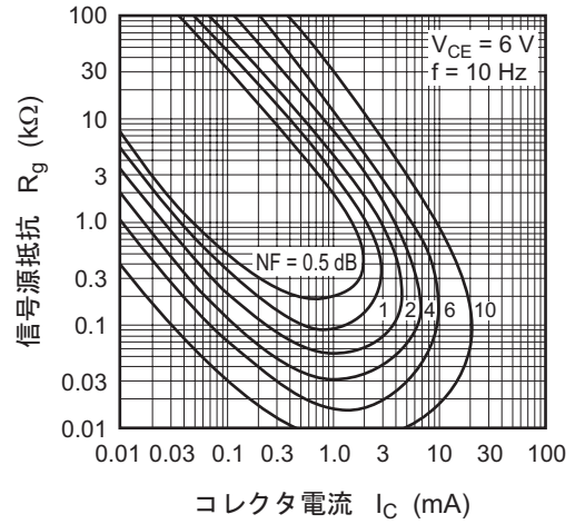
雑音特性
