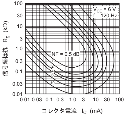
雑音特性
